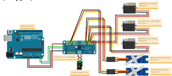
Gambar 4. Rancangan Elektronik
