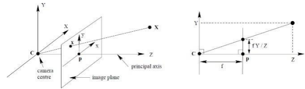
Gambar 1. Pinhole Kamera
