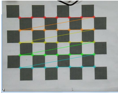
Gambar 7. Proses Kalibrasi
