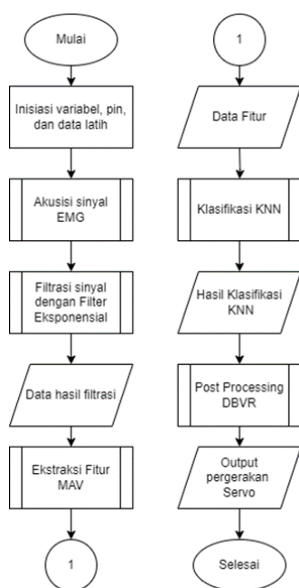
Gambar 4. Diagram Alir Sistem
