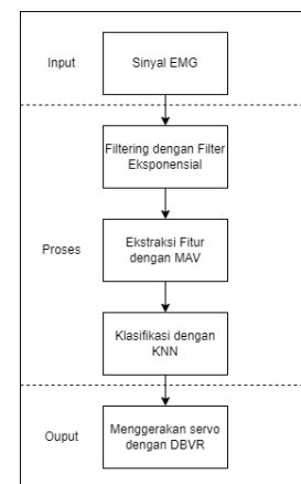
Gambar 1. Blok Diagram Sistem
