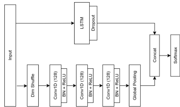
Gambar 6. Arsitektur LSTM-FCN Modifikasi
