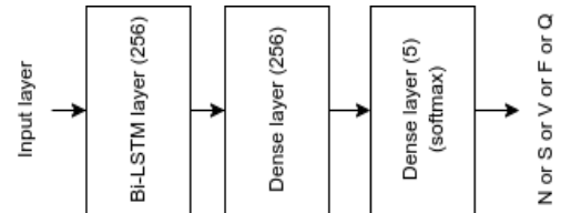
Gambar 5. Arsitektur Bi-LSTM
