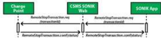
Gambar 7 Skema Aliran Data Menghentikan Pengisian Daya
