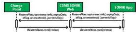
Gambar 11 Skema Aliran Data Memulai Proses Reservasi
