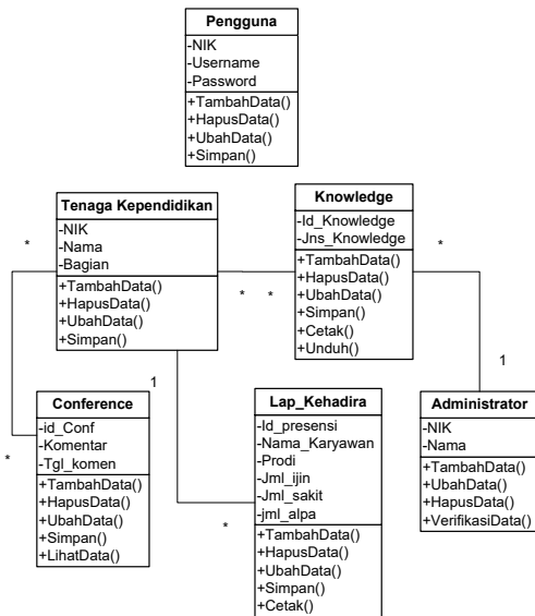
Gambar 8. Class Diagram KMS Fakultas Teknik
